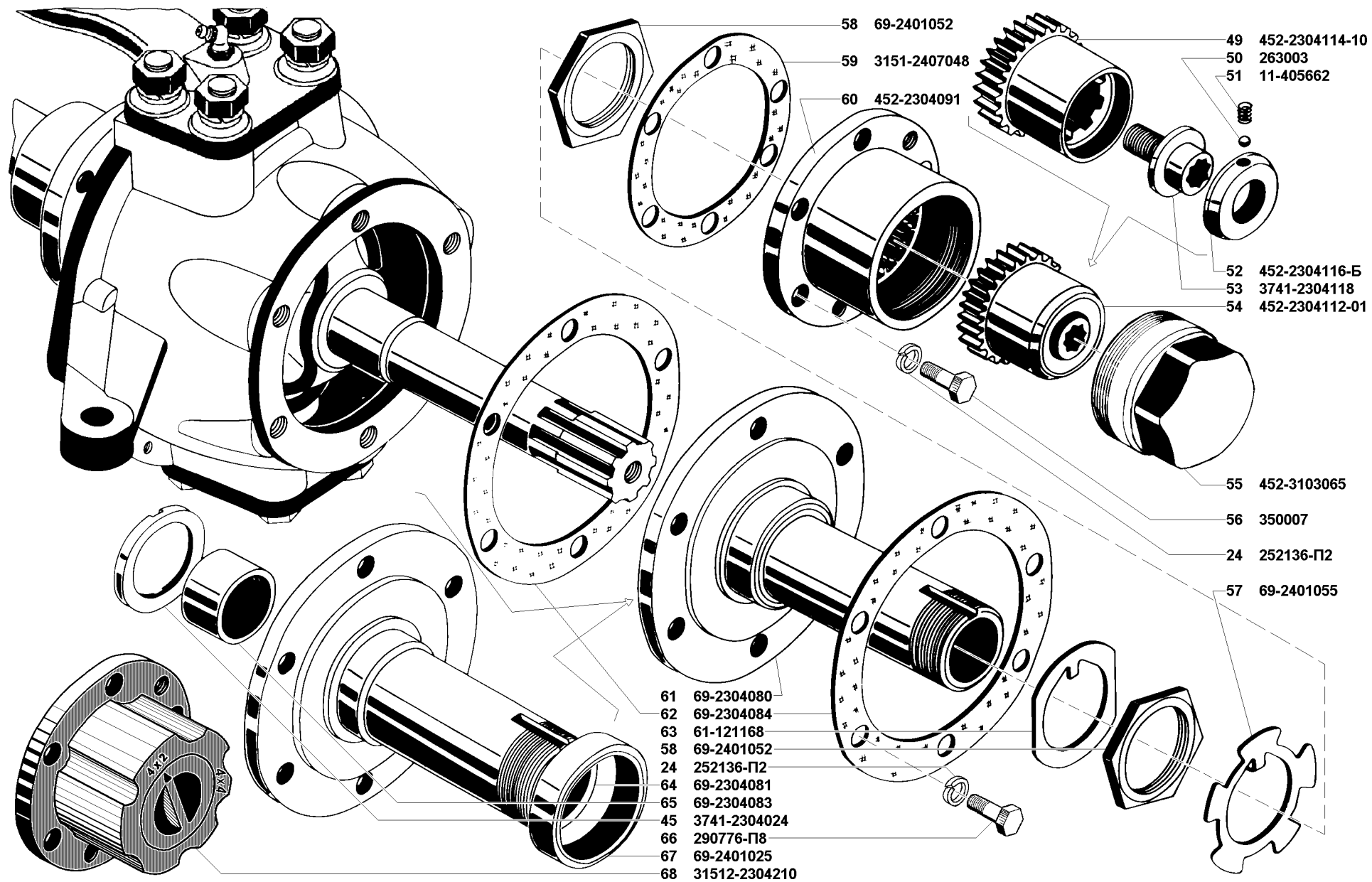
Рис. 62. Кулаки поворотные (2304)/3
